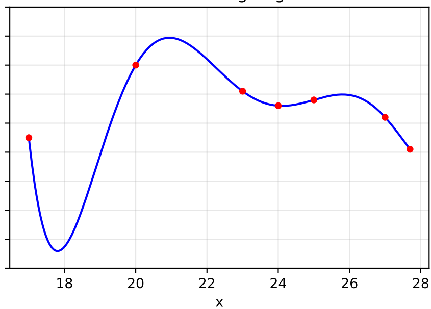
Curva 2: Lagrange
